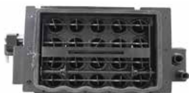
pulizia automatica fascio tubiero vista dall'alto
